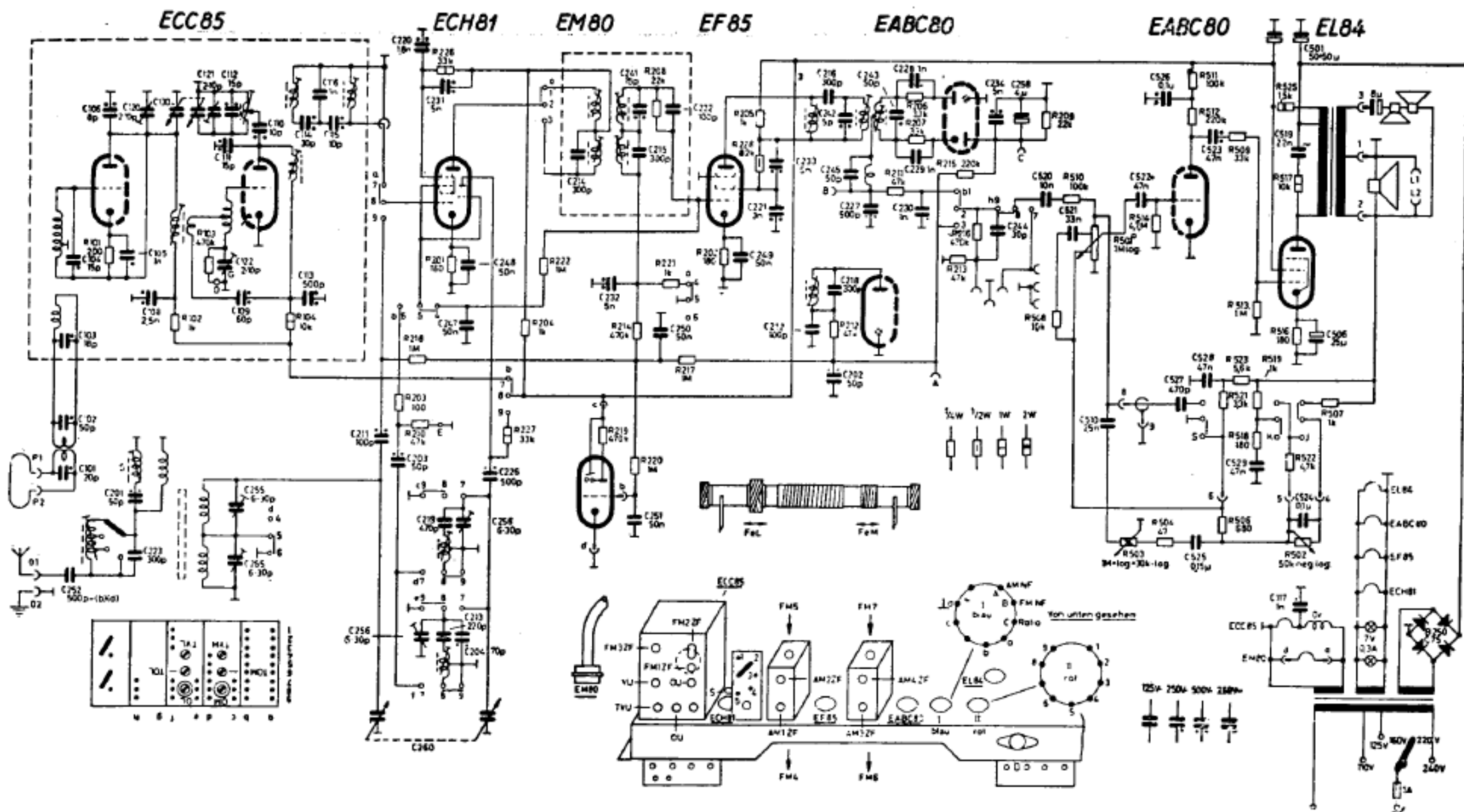
METZ RADIO APPARATEFABRIK (Capriotti) - Mod. AM/FM 308. A modulazione d'ampiezza e di frequenza. Onde lunghe, medie, corte e ultracorte (FM). Media frequenza AM a 460 kc/s, FM a 10,7 Mc/s. Antenna interna in ferrite. Tre altoparlanti. Potenza 4 watt indistorti. Consumo 45 watt.
